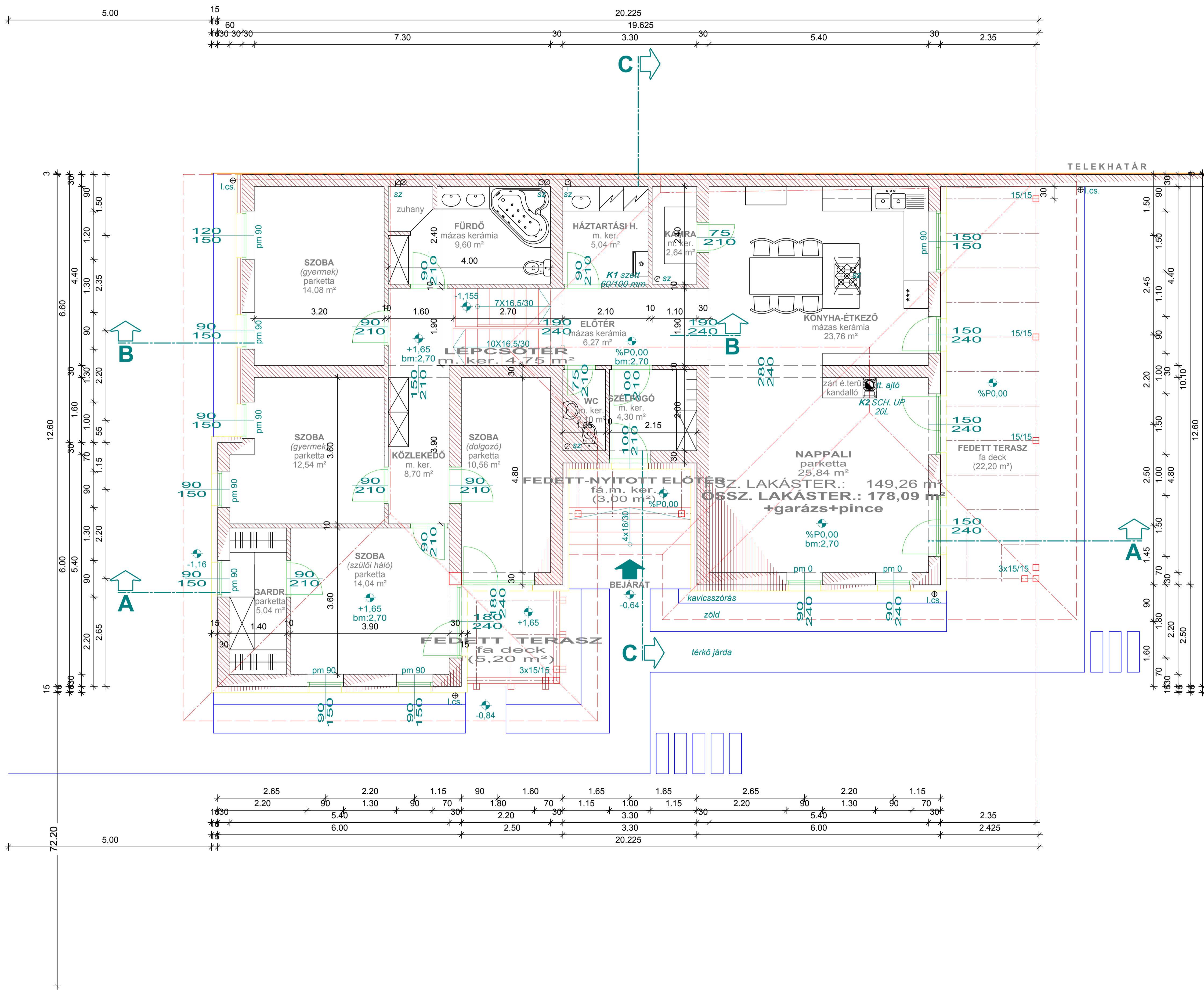
45 SORSZÁM CSALÁDI HÁZ FELMÉRÉSI (EREDETI) ALAPRAJZ 1:50
